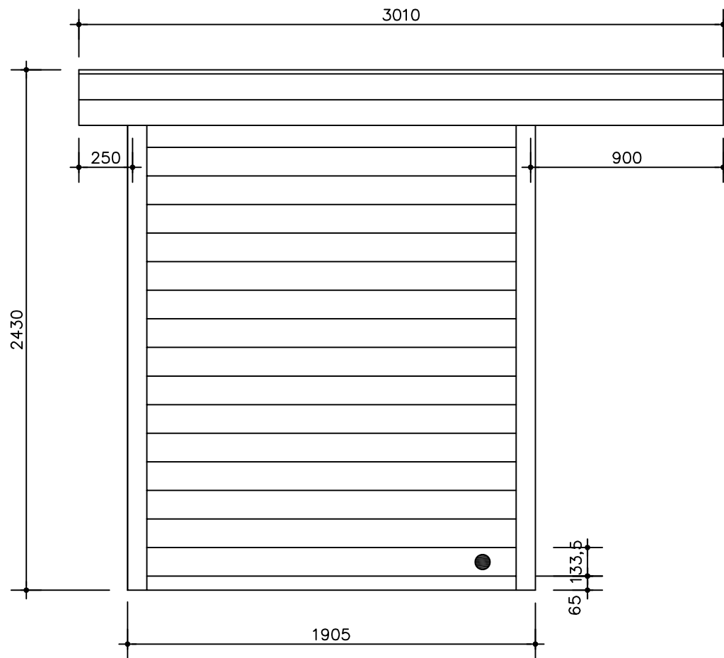
Zijaanzicht links
