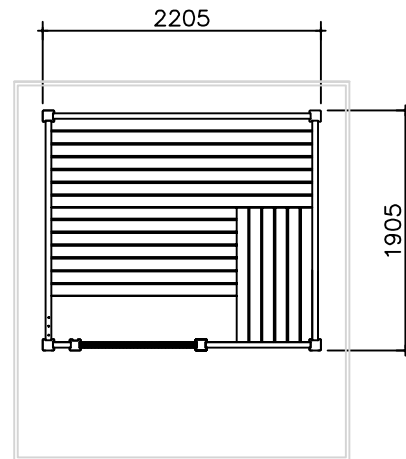
Grondplan
