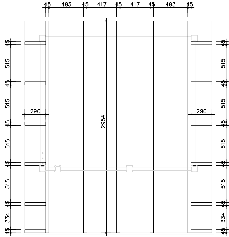
Legplan dakbalken
