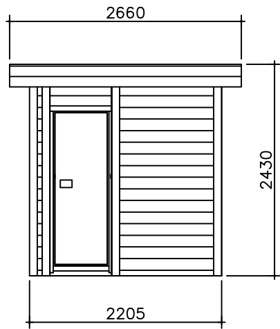
Vooraanzicht
