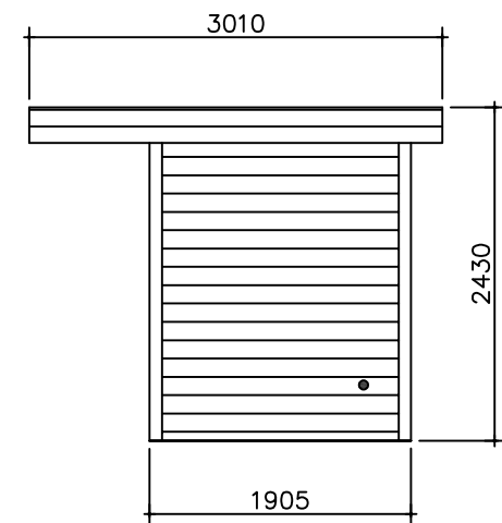
Zijaanzicht rechts
