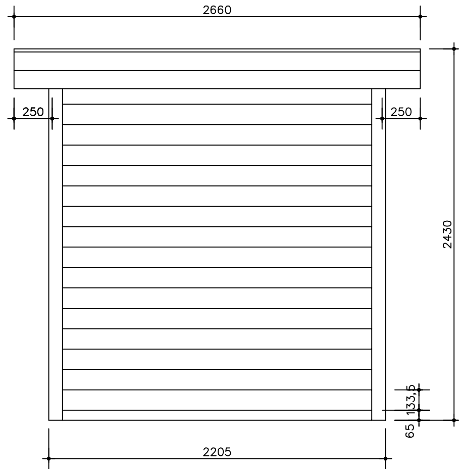
Achteraanzicht
