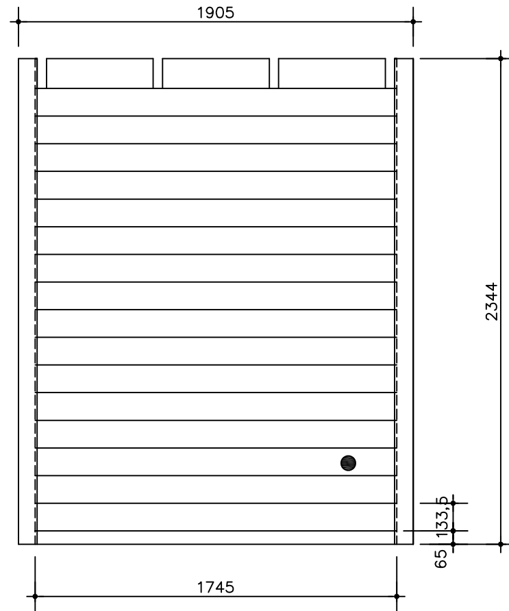
Zijaanzicht rechts
