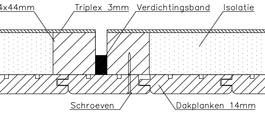
Detail dakconstructie
