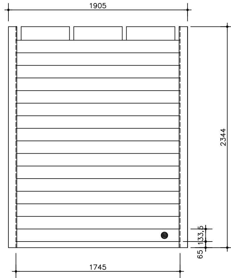
Zijaanzicht links
