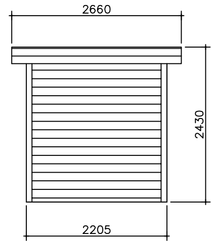
Achteraanzicht
