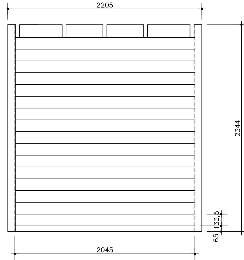
Achteraanzicht
