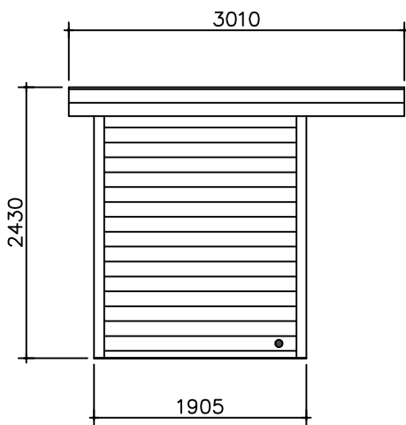
Zijaanzicht links
