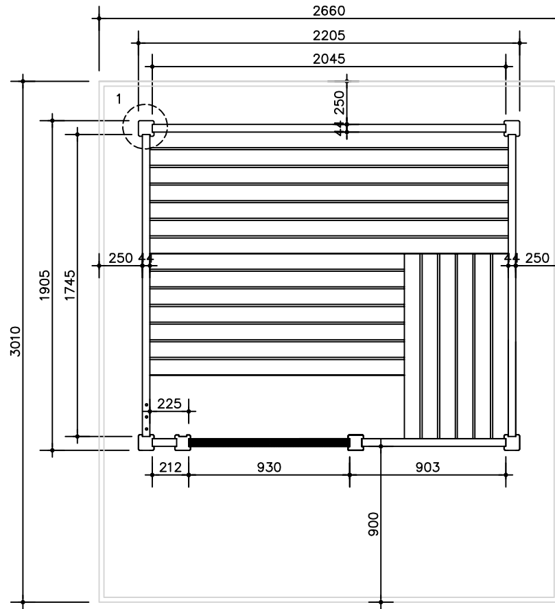
Grondplan
