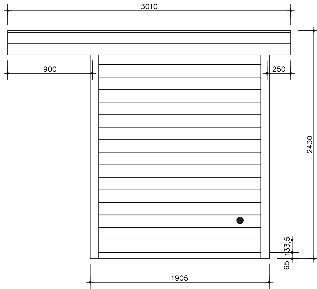
Zijaanzicht rechts
