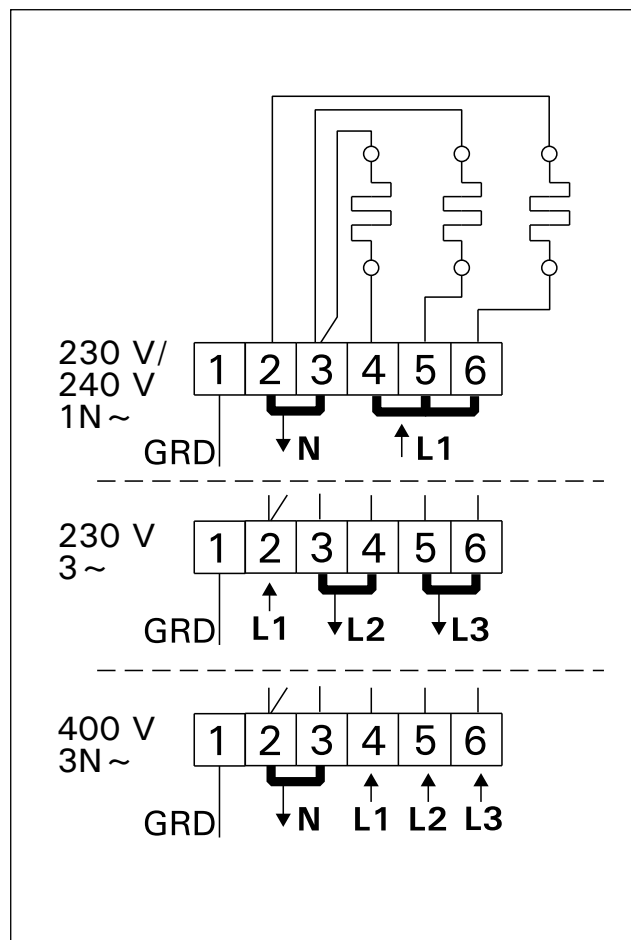
Рисунок 11. Электромонтаж каменки BC-E Joonis 11. BC-E-kerise elektrühendused
